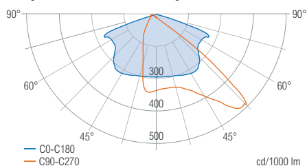
Schrägbreitstrahlende Lichtverteilung
